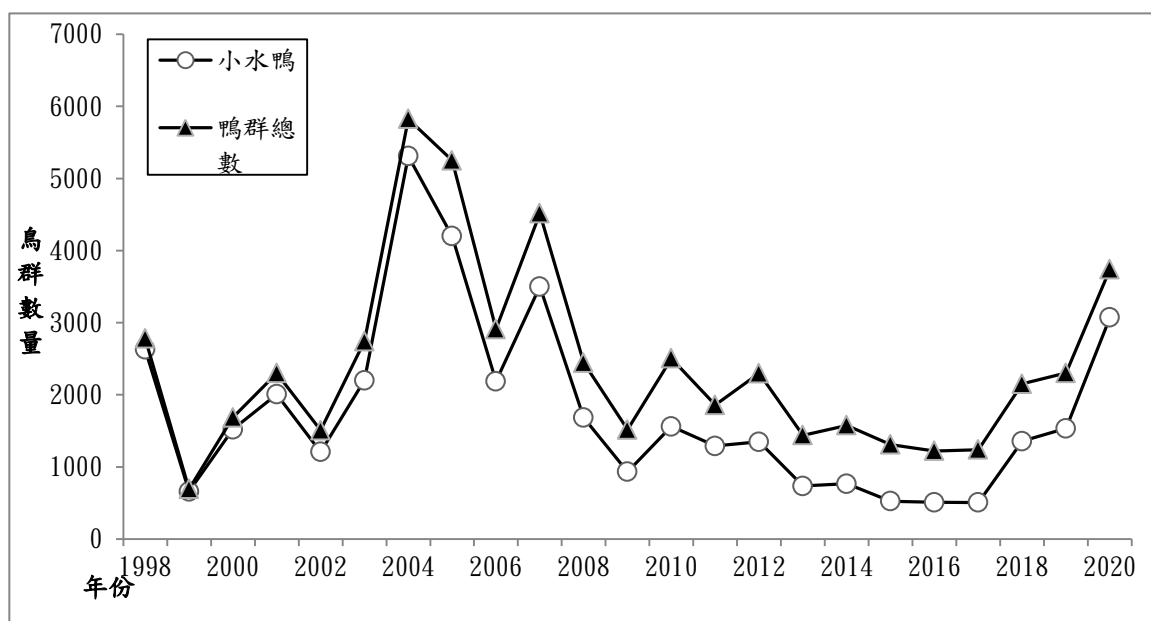
▲1998 至 2020 年關渡自然公園穿越線鳥調的鴨群及小水鴨數量變化。
